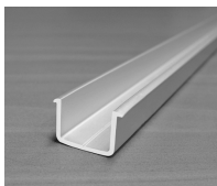
01103.DN80.PG - Guía inferior embutida 3 mt. Mecanización 21 mm. ancho 15 mm. profundidad Embalaje: 1 ud.
