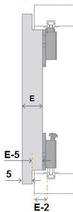
MONTAJE MIXTO
