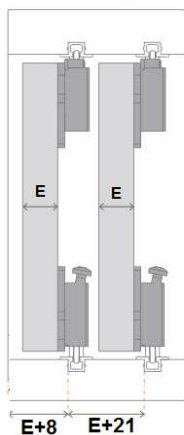
MONTAJE EMBUTIDO
