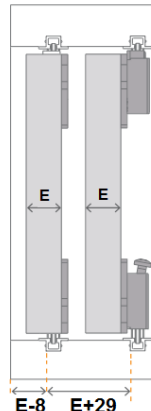
MONTAJE MIXTO
