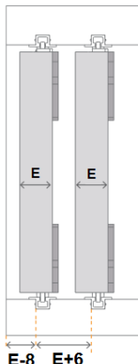
MONTAJE EMBUTIDO
