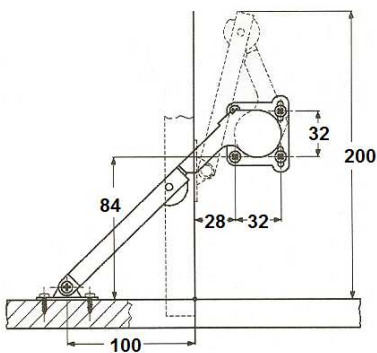
00701.0601 - Puerta abatible Compás descendente niquelado Con freno regulable Mano: izquierda-derecha Embalaje: 1 / 10 uds.
