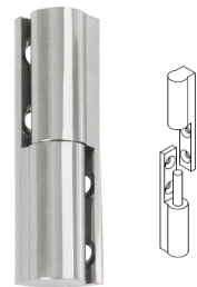
00206.0694.L - Dorado brillo 00206.0694.N - Níquel brillo Bisagra con pasador Material: latón Dimensiones: 50x10 mm. Embalaje: 1 / 100 uds.
